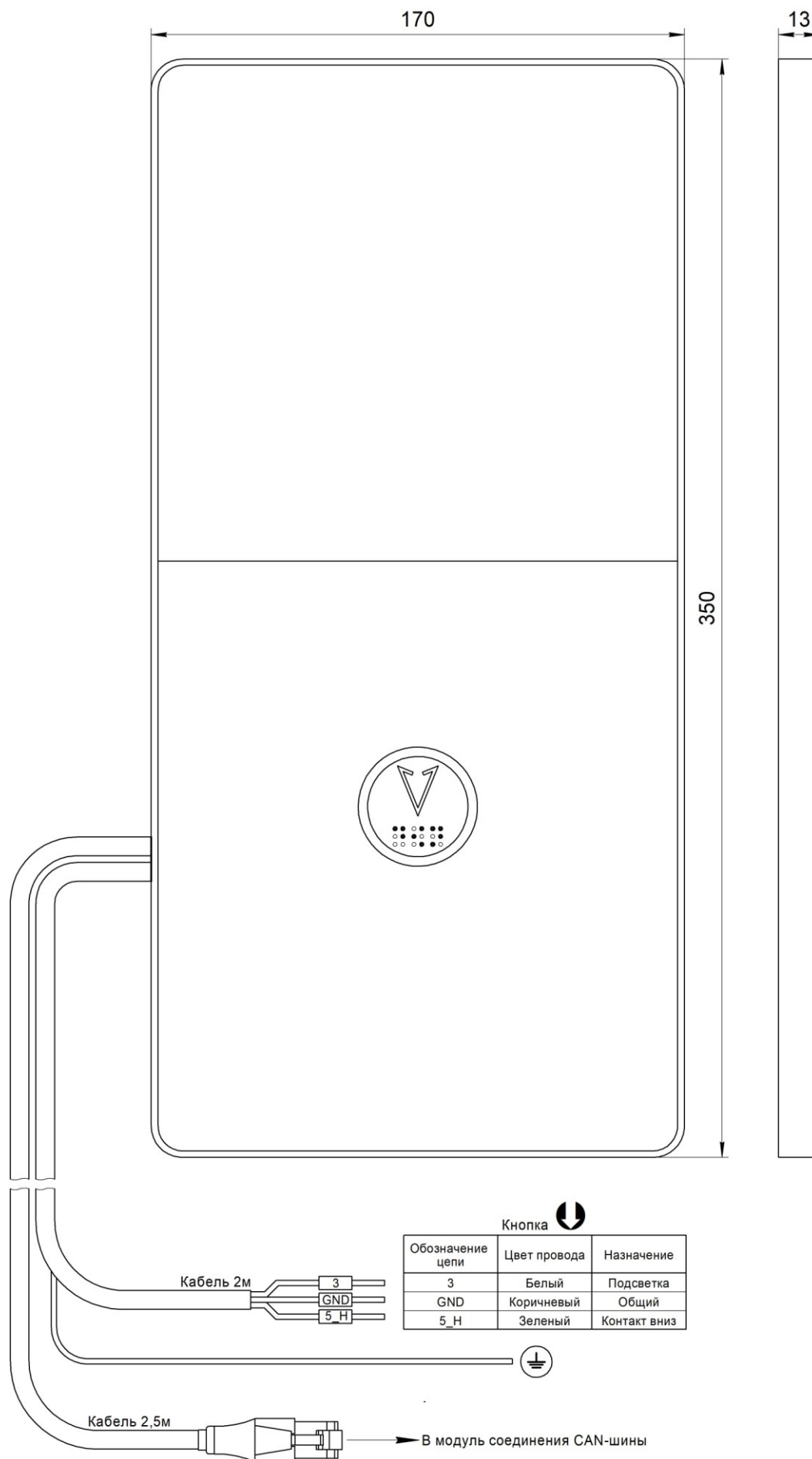
Рис.1 Внешний вид, габаритные и установочные размеры Вызывного поста МАЛАХИТ (жгут RJ45) НШЕК.468381.017-01
